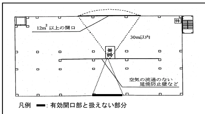
《車室の各部分から水平距離30m以内の外周部の12㎡以上の有効開口部の例》
