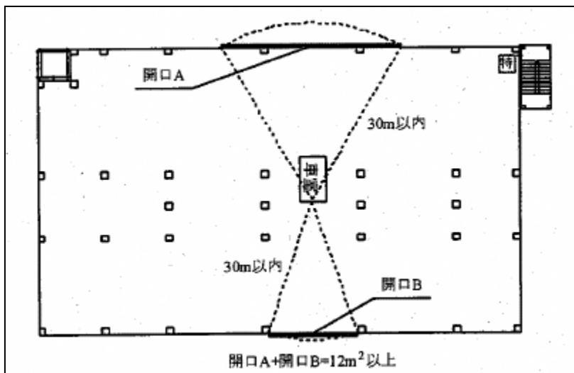
《車室の各部分から水平距離30m以内の外周部の12㎡以上の有効開口部の例》
