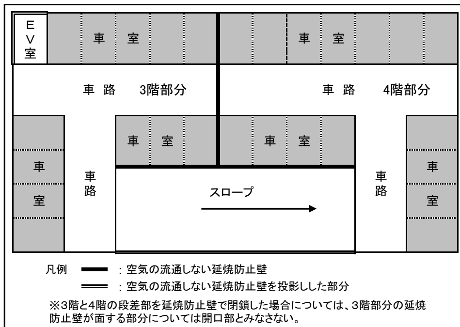
《フラット段差式の自走式駐車場開口部の判断の例》
